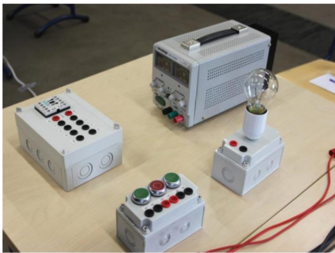
Kytkentätehtävä → lamppu syttyy
